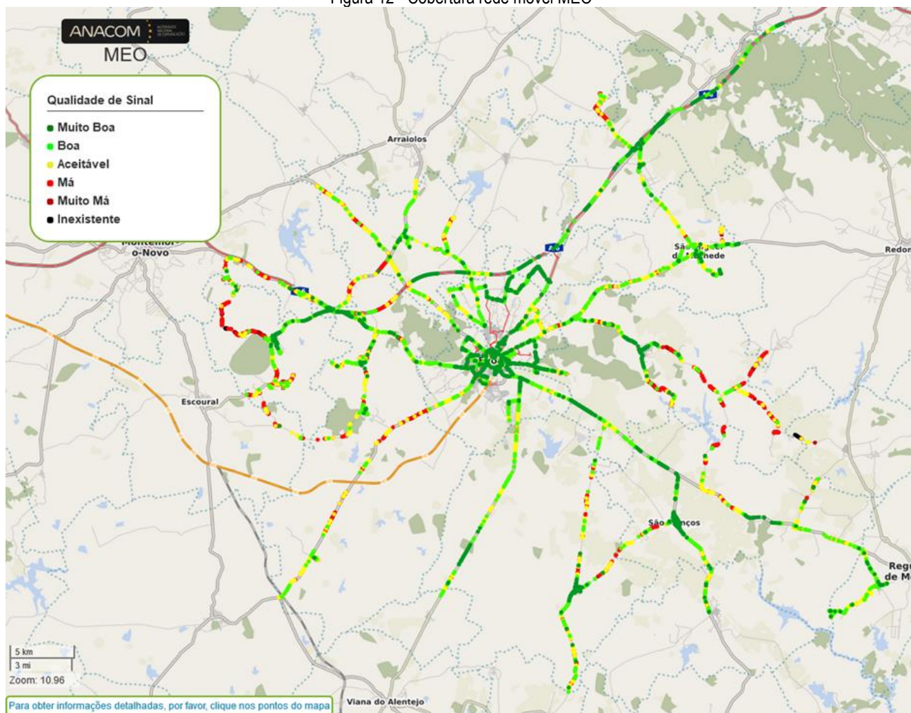
Figura 12 - Cobertura rede móvel MEO
