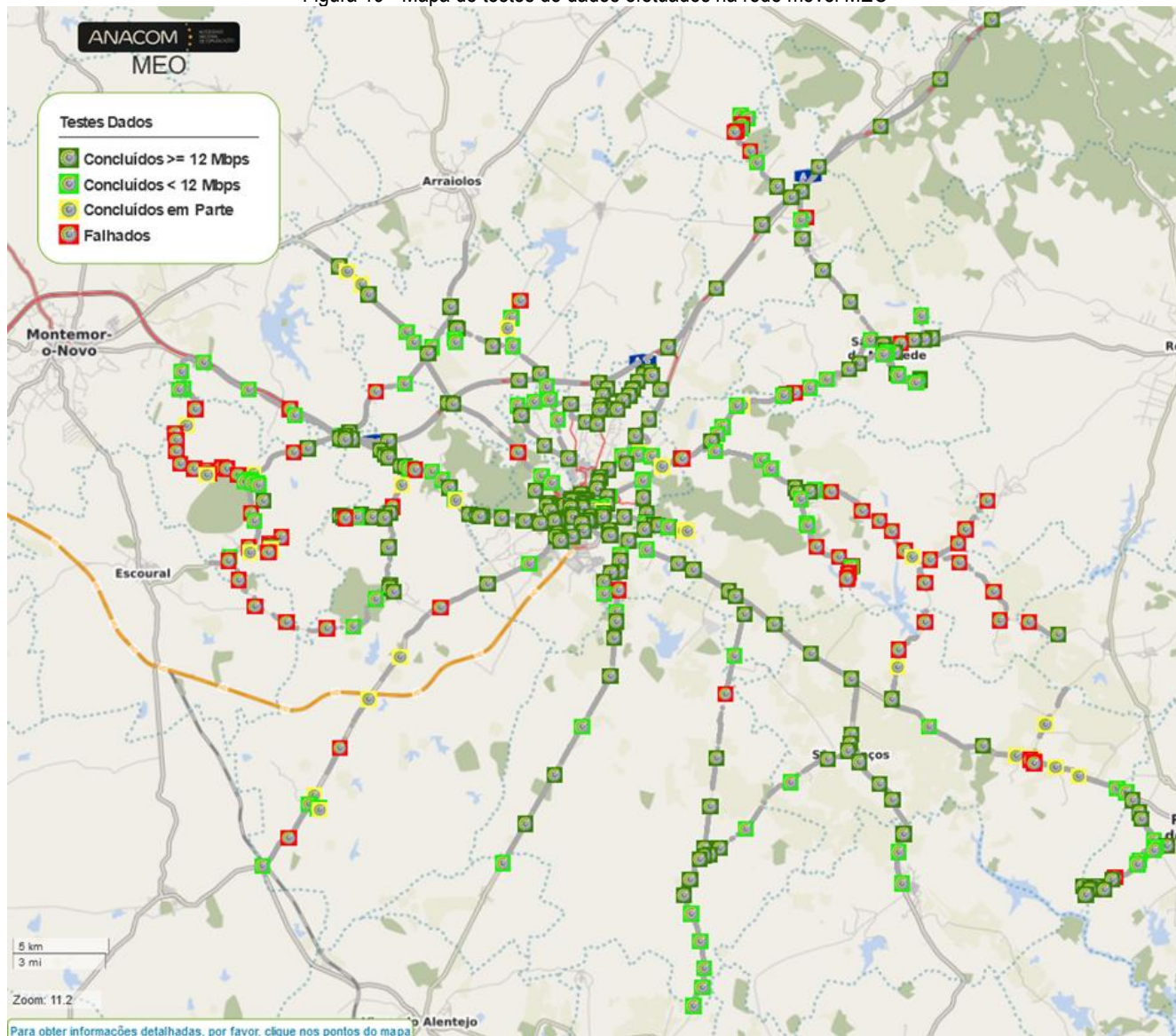
Figura 19 - Mapa de testes de dados efetuados na rede móvel MEO
